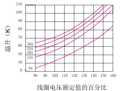
线圈温升
