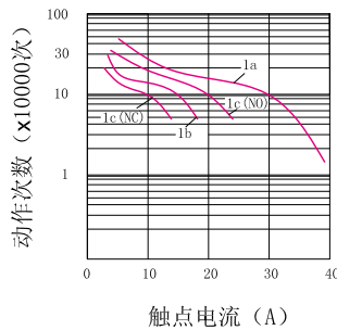
寿命曲线
