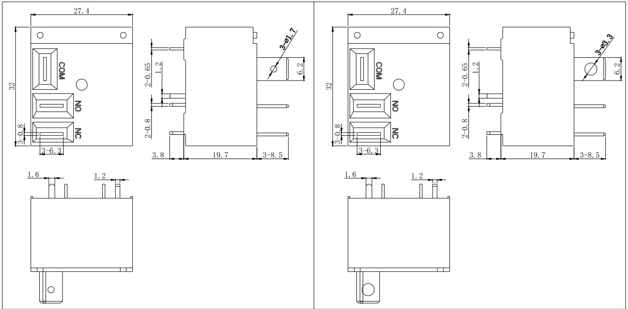
小吊孔外形图
