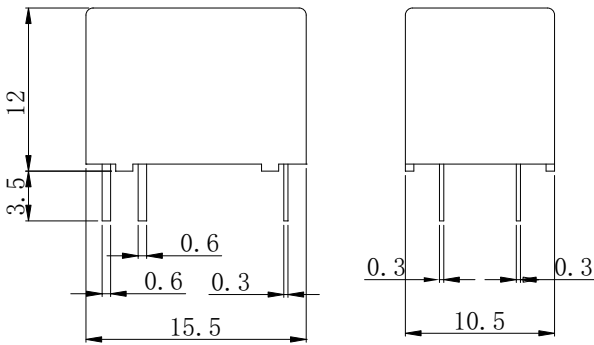
外形图
